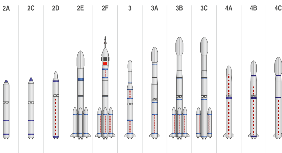
Abb. 3: Von DF-5 abgeleitete Raumfahrtträger „Langer Marsch“
